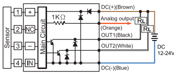
KP4□0 - 010 2 NPN + Analog Output (1~5V)
