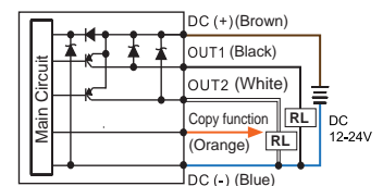
KP43 □ - 04 - □ 2 PNP + Copy Function
