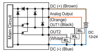
KP43 □ - 031 - □ 2 PNP + Analog Output(4~20mA)
