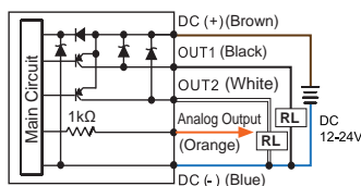
KP43 □ - 030 - □ 2 PNP + Analog Output(1~5V)
