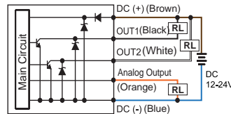
KP43 □ - 011 - □ 2 NPN + Analog Output(4~20mA)
