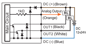
KP43 □ - 010 - □ 2 NPN + Analog Output(1~5V)
